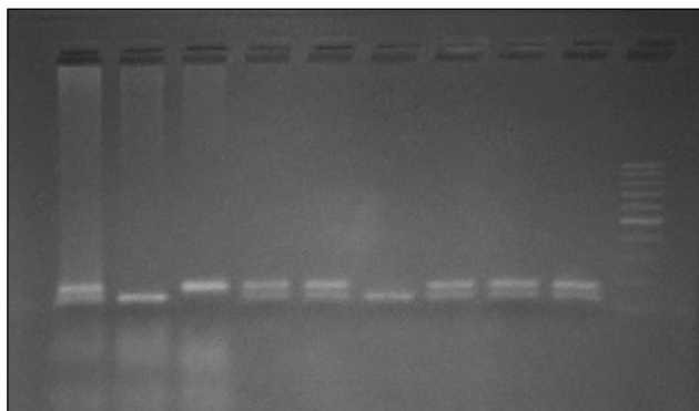
Рис. 1. Электрофореграмма продуктов гидролиза амплификатов участка гена CSN2 эндонуклеазой рестрикции BstDEI
